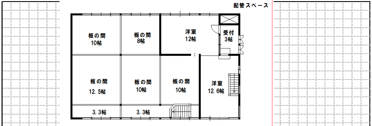
2階平面図
